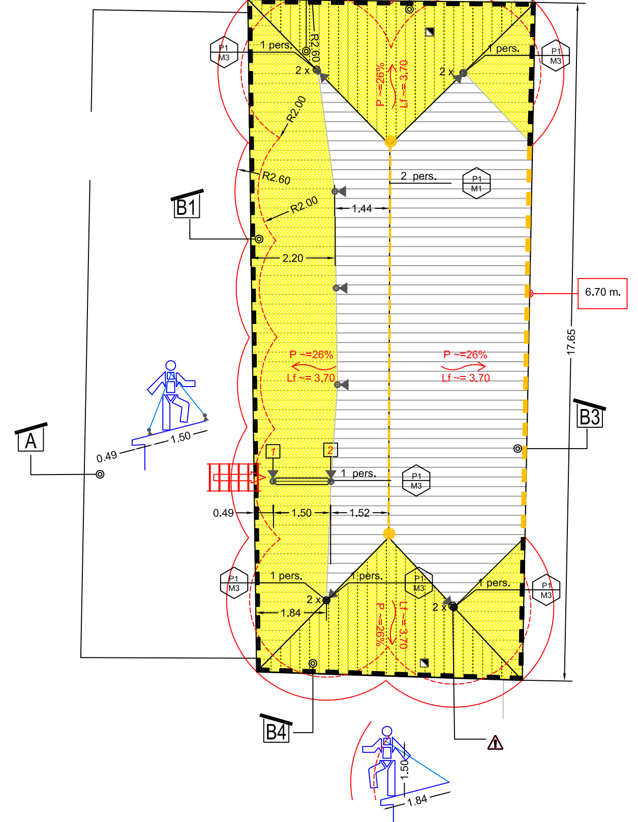
Pianta Copertura
